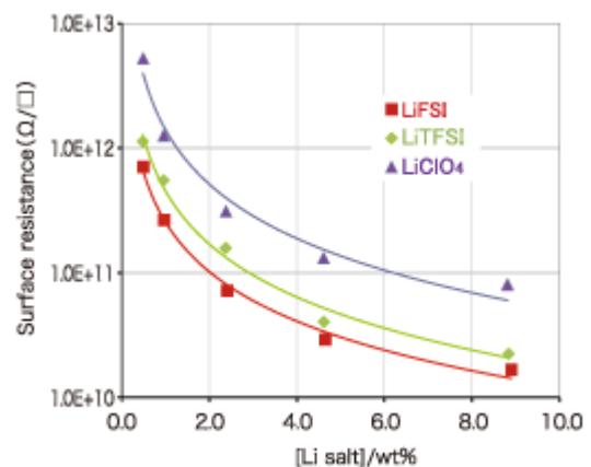
그림 5. LiFSI의 정전기 방지효과가 LiTFSI, LiClO4 대비 우수하다
