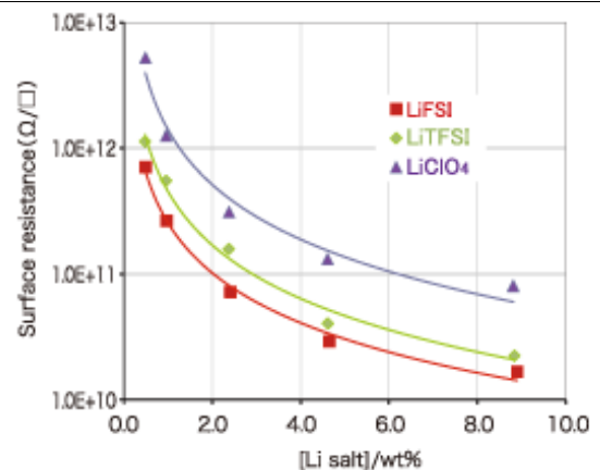
그림 48. LiFSI 의 정전기 방지효과가 LiTFSI, LiClO 4 대비 우수
