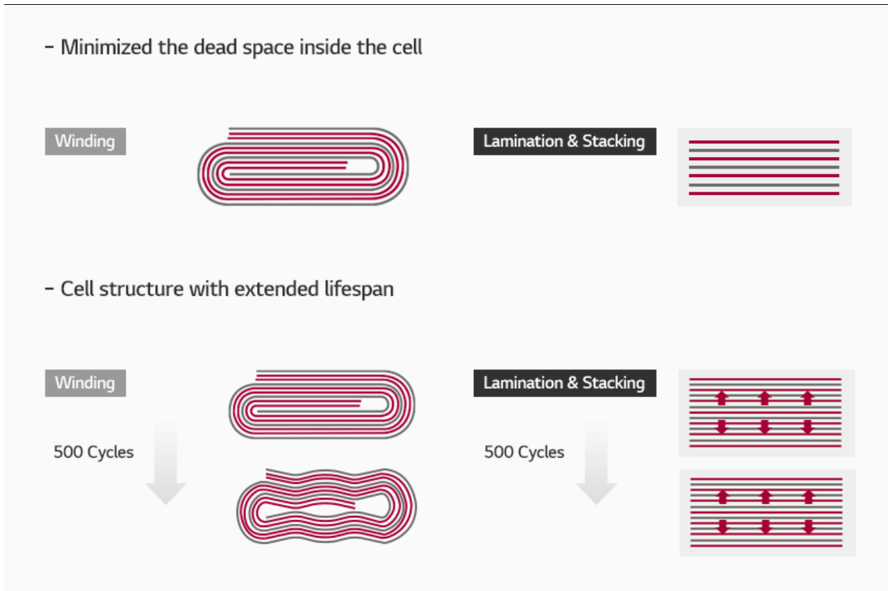
그림 66. 배터리 내부 소재 생산 공정인 Winding 방식과 Stacking 방식 장단점 비교
