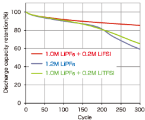
그림 2. 300 회의 충방전을 반복하였을때, 순수하게 LiPF6만 추가된 배터리의 경우 충방전능력이 설계용량 대비 60% 수준으로 감소하는 반면에, LiFSI를 추가하면 80% 이상으로 유지됨을 확인할 수 있다.
