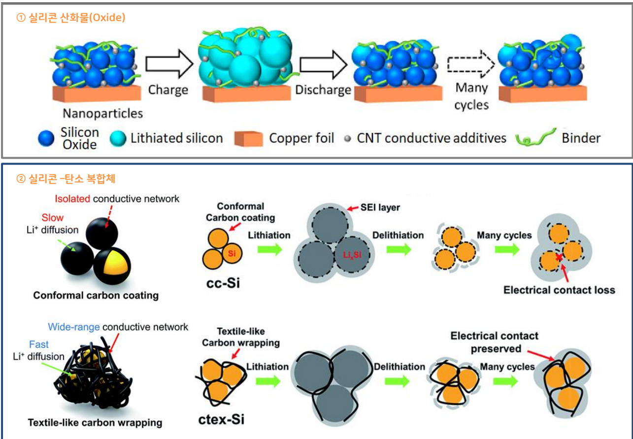
그림 34. 대표적인 실리콘 음극활물질 적용 기술인 실리콘 산화물과 실리콘-탄소 복합체 방식 비교
