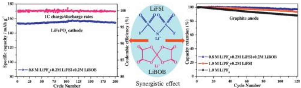
그림 55. LiPF 6 에 더해 LiFSI와 LiBOB를 혼용하였을 때, LiPF 6 및 LiPF 6 /LiFSI 혼용 배터리 대비 수명이 증가하였음을 확인
