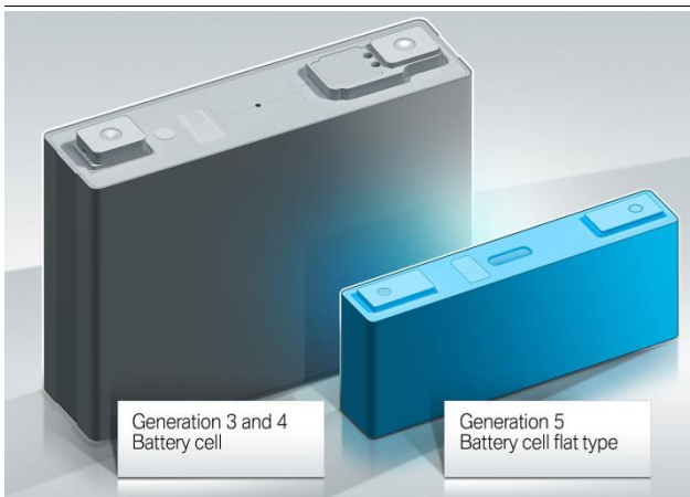
그림 64. 2021 년 BMW 로 공급될 삼성 SDI Gen5 중대형 배터리
