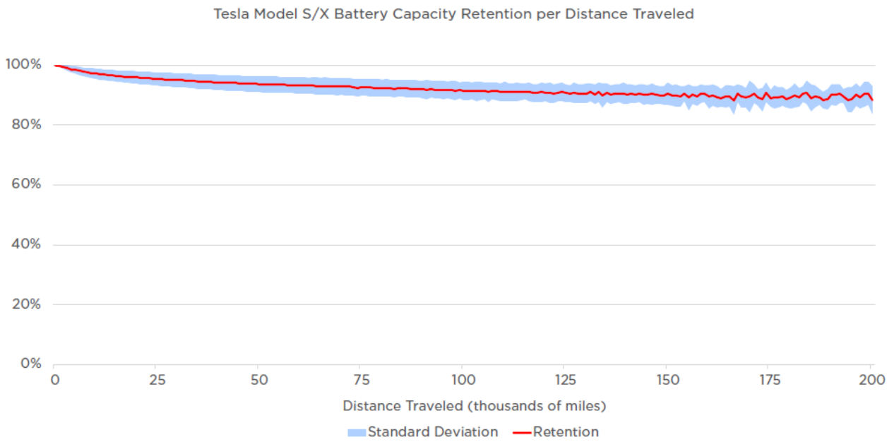
그림 13. 테슬라 Model S/X 주행거리에 따른 배터리 용량 유지율(수명) 추이
