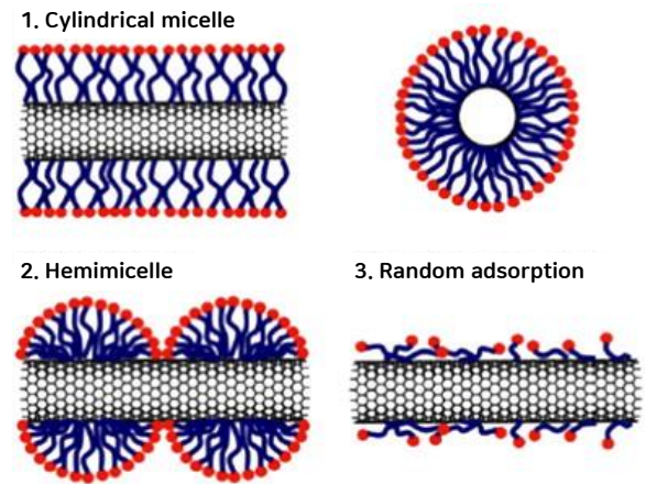
그림 6. 계면활성제를 활용한 CNT(탄소나노튜브) 분산법
