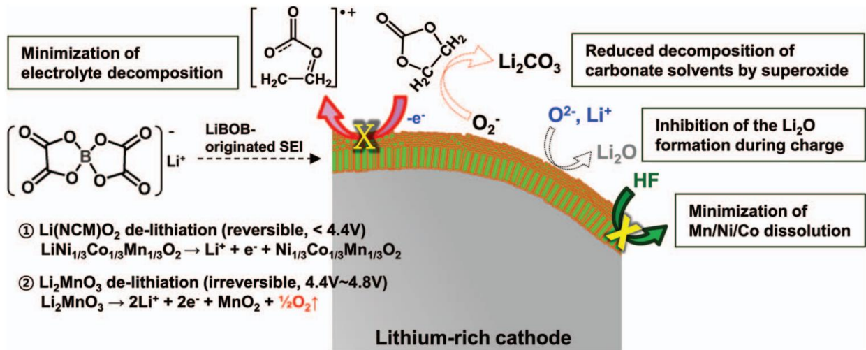
그림 54. LiBOB 추가에 따른 SEI 형성으로 인해 ① 전해질 분해가 억제되며, ② 활성 산소에 의한 용매 분해가 억제되고, ③ 충전시의 산화리튬 형성을 방지하며, ④ 망간/니켈/코발트의 용해 억제
