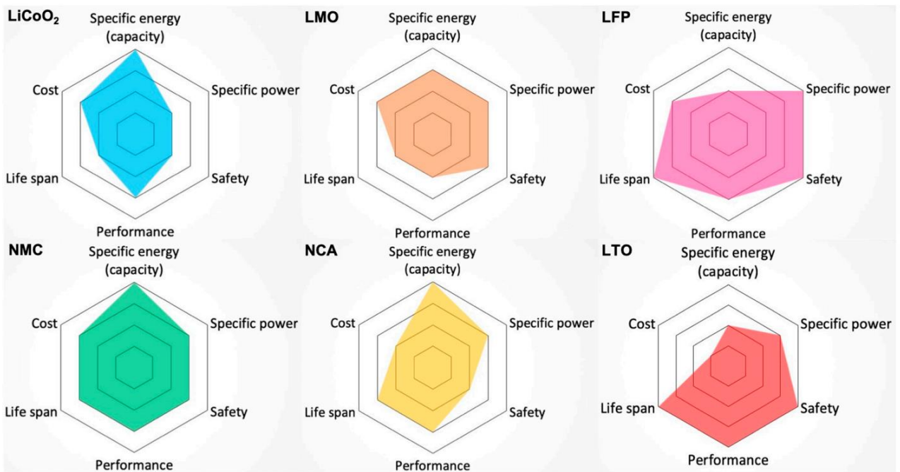
그림 22. 주요 양극활물질 소재별 장단점 비교
