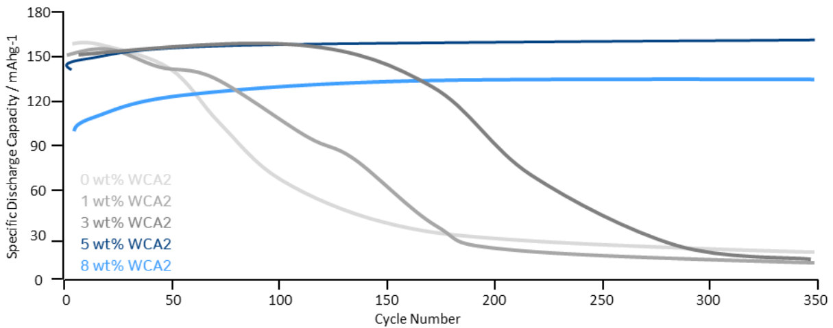
그림 52. LiPF 6 에 더해 LiDFOB(WCA2)를 첨가하였을 때 배터리 수명이 급격히 개선되는 모습을 확인
