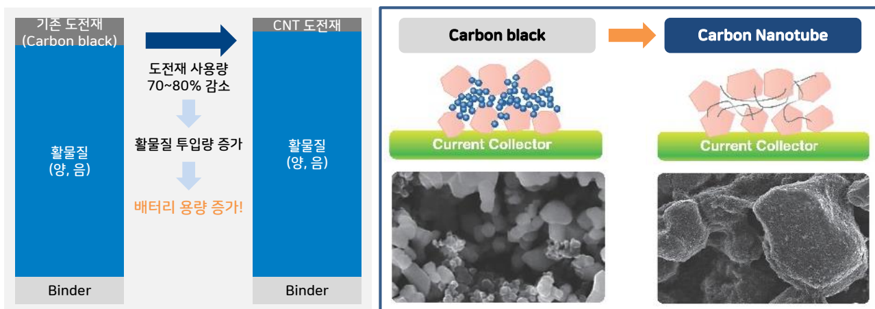
그림 42. 양극재에 CNT 도전재를 사용할 경우 도전재 사용량을 1/5 로 줄일 수 있어 체적 에너지 밀도 향상
