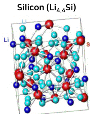
그림 31. 실리콘은 실리콘 원자 1 개당 리튬이온 4.4 개를 저장
