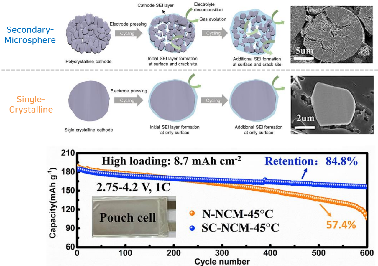
그림 19. 단결정 양극재는 부서지는 잔해물과 불순물이 없기 때문에 수명 향상, 에너지 밀도 증가, 가공비 절감 등의 효과 기대
