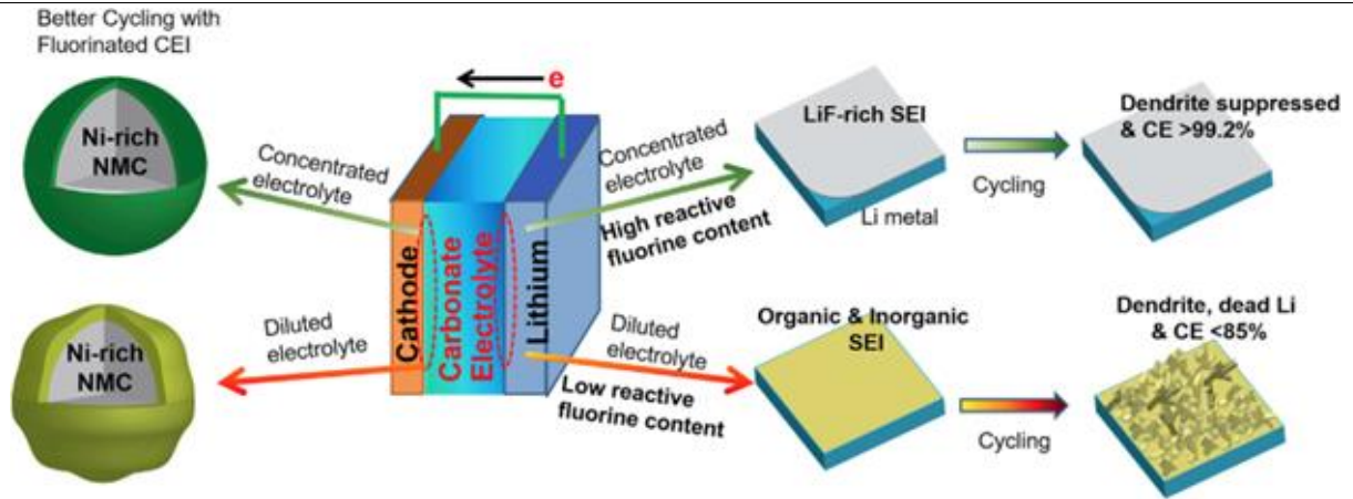
그림 1. LiFSI의 FSI 음이온은 리튬양극과 반응해 LiF-rich SEI를 형성하며, 결과적으로 덴드라이트 발생 확률을 극적으로 낮춘다.
