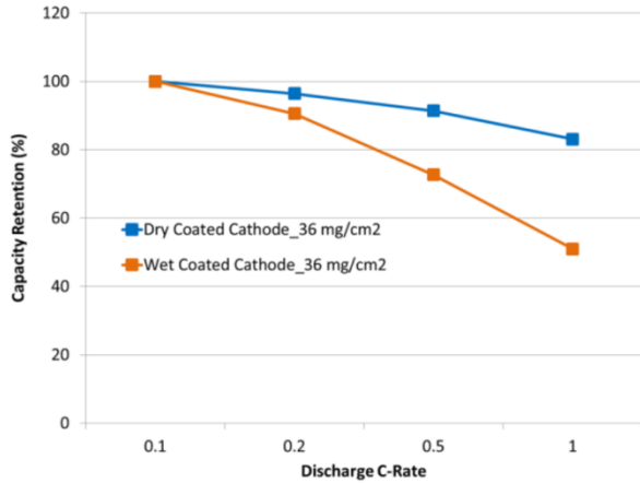
그림 4. 건식/습식 전극 코팅방식 배터리 용량 유지율(수명) 비교
