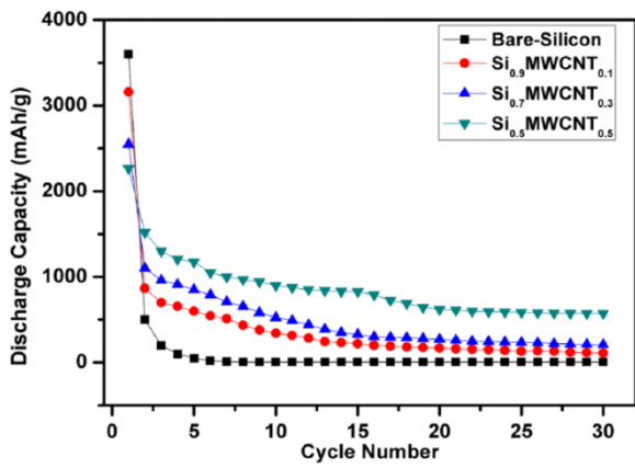
그림 35. 실리콘 음극재와 CNT 도전재 적용시 에너지 용량 증가
