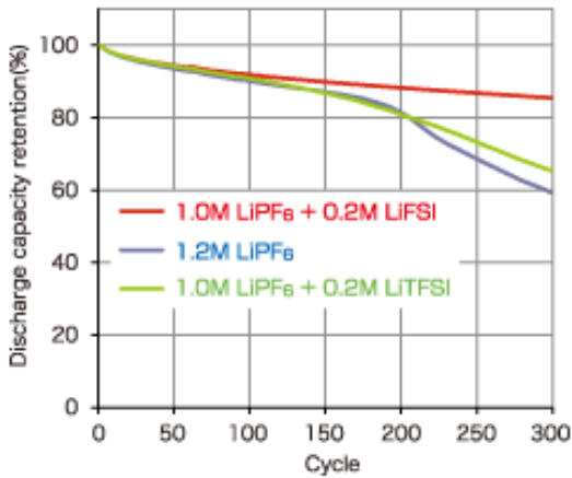
그림 46. LiPF 6 만 추가된 배터리 경우 충방전능력이 설계용량 대비 60% 수준으로 감소하는 반면, LiFSI 추가시 80% 이상으로 유지
