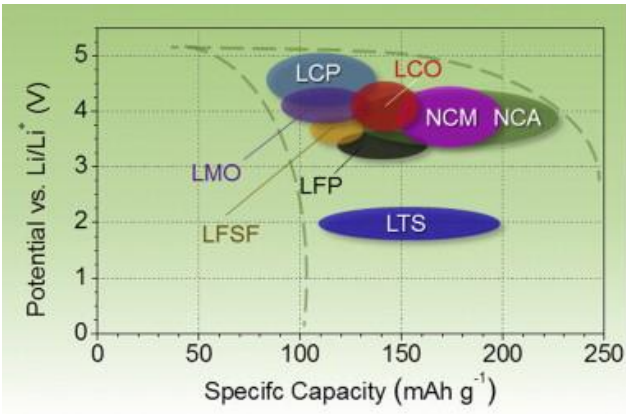
그림 20. 주요 양극활물질 종류별 에너지 용량 비교
