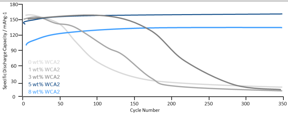
그림. LiPF 6 에 더해 LiDFF(WCA2)를 첨가하였을 때 배터리 수명이 급격히 개선되는 모습을 확인할 수 있음
