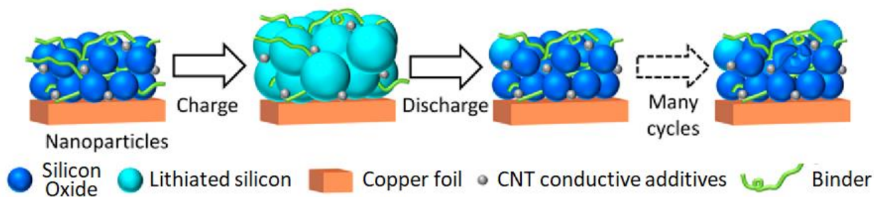
그림 44. CNT 도전재가 실리콘 음극재의 팽창을 잡아주는 보완재로서 중요성 부각
