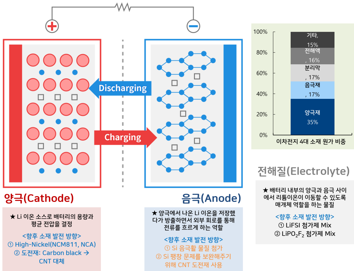
그림 27. 리튬 배터리의 구조와 주요 소재별 첨가제 기술 변화 전망
