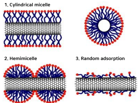
그림 41. 계면활성제를 활용한 CNT(탄소나노튜브) 분산법
