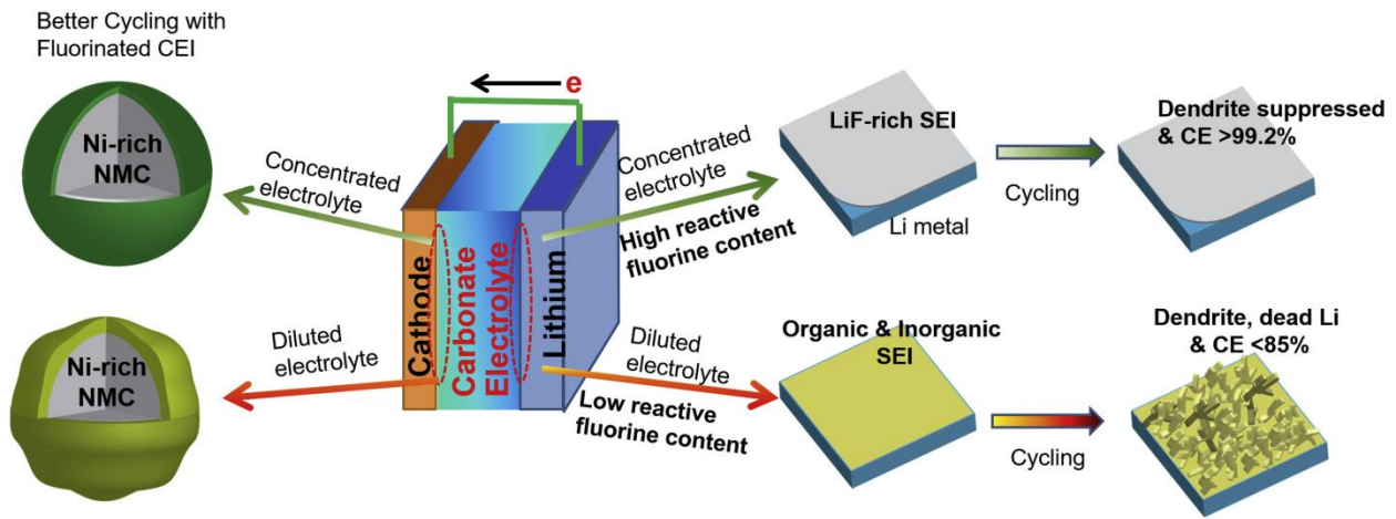
그림 45. LiFSI 의 FSI 음이온은 리튬 양극과 반응하여 LiF-rich SEI 를 형성하며, 결과적으로 Dendrite 발생 확률을 극적으로 완화
