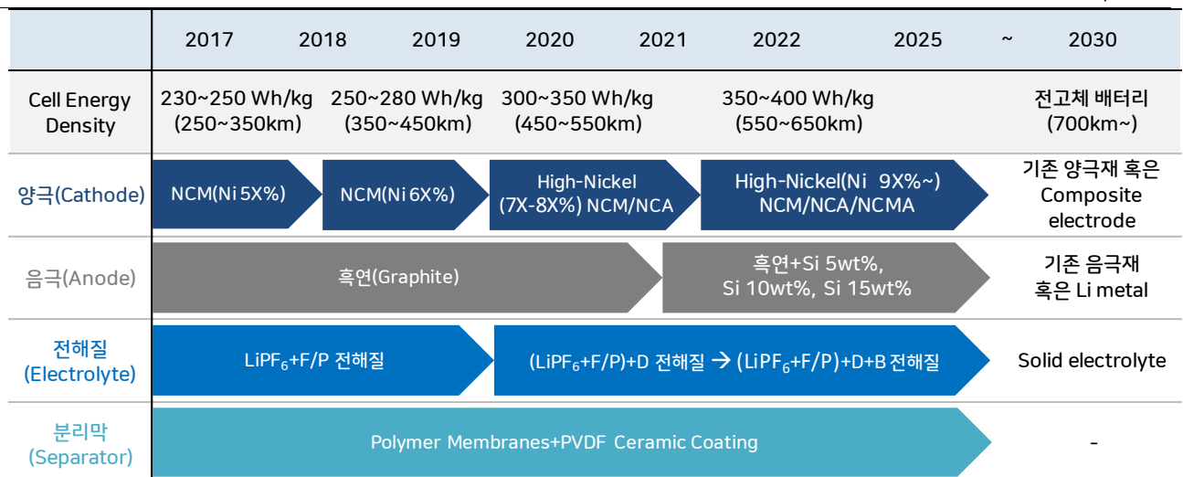
그림 3. 주요 배터리 업체들의 '에너지밀도 향상, 수명 개선, 충전시간 단축, 저온성능 개선'을 위한 주요 소재별 기술 변화 Road-map
