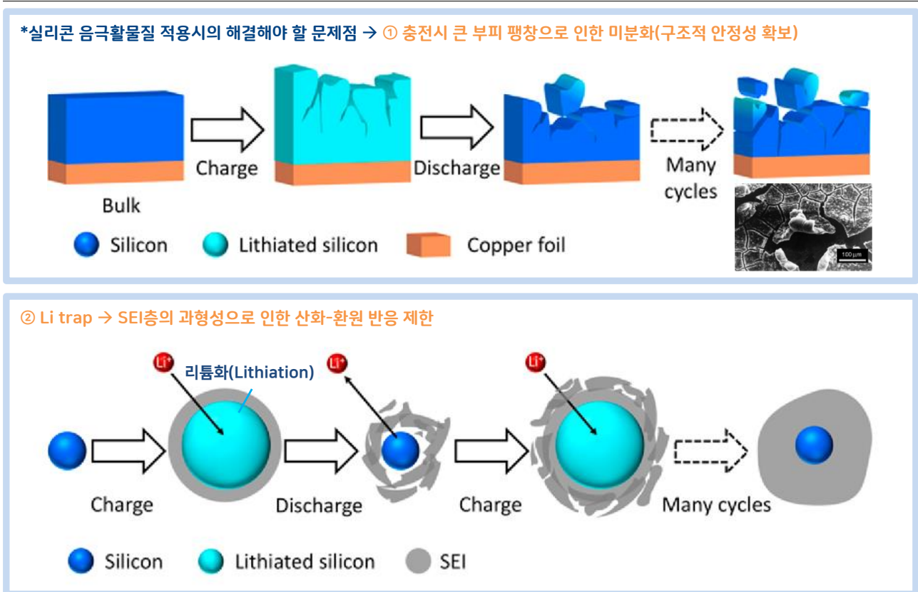
그림 33. 실리콘 음극활물질의 문제점 - 1. 구조적 안정성, 2. 실리콘 리튬화에 따른 SEI층의 과형성
