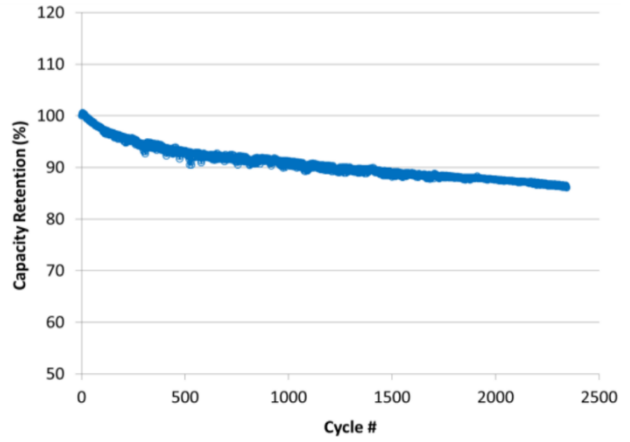
그림 5. Maxell 습식전극 코팅방식 배터리 충방전 Cycle(수명) 실험
