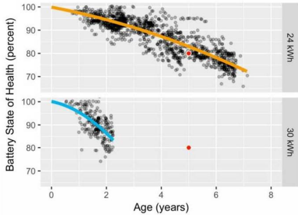
그림 14. Nissan Leaf 의 사용연수에 따른 배터리 성능저하 상태표
