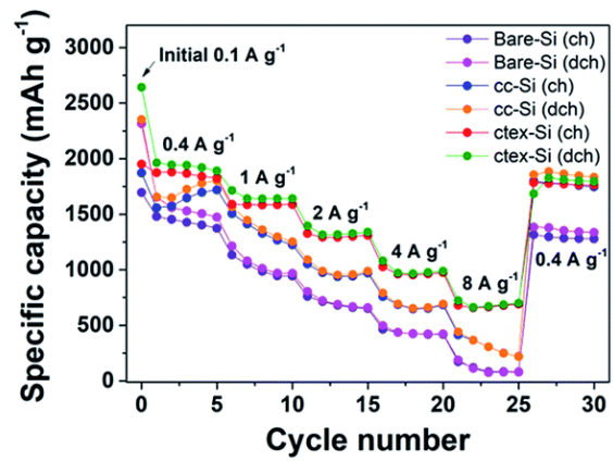
그림 36. 실리콘-탄소 복합체로 음극재 적용시 에너지 용량 증가
