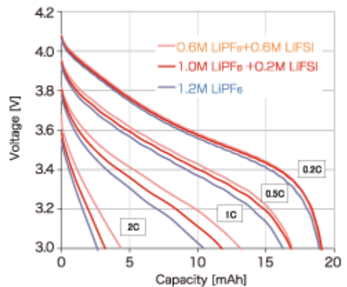
그림 3. -20°C의 저온에서 테스트 하였을때, LiFSI를 전해질로 첨가한 배터리의 방전 억제율이 LiPF6만 추가된 배터리 대비 높다
