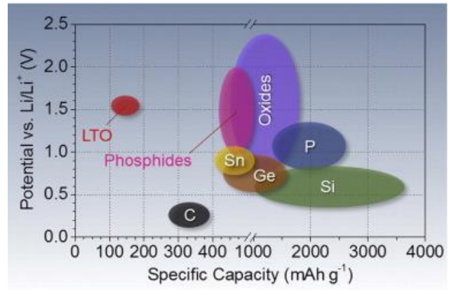
그림 21. 주요 음극활물질 종류별 에너지 용량 비교
