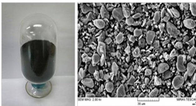
그림 39. 대주전자재료의 Mg-SiO 음극활물질
