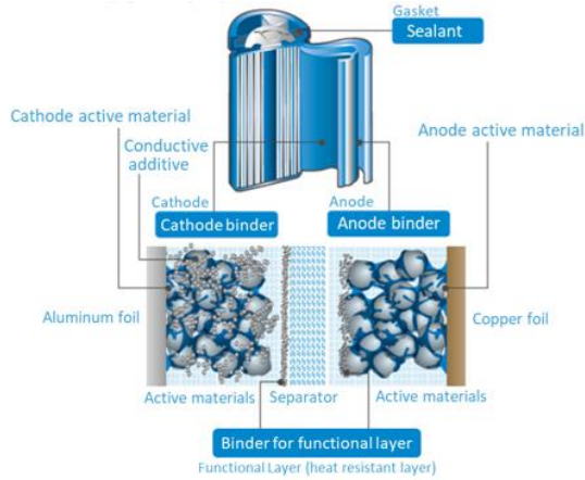
그림 1. 리튬이온전지 Binder 종류 및 구조
