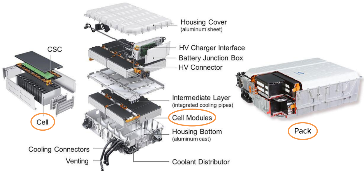
그림 24. 전기차 중대형 배터리 Cell → Module → Pack 구조
