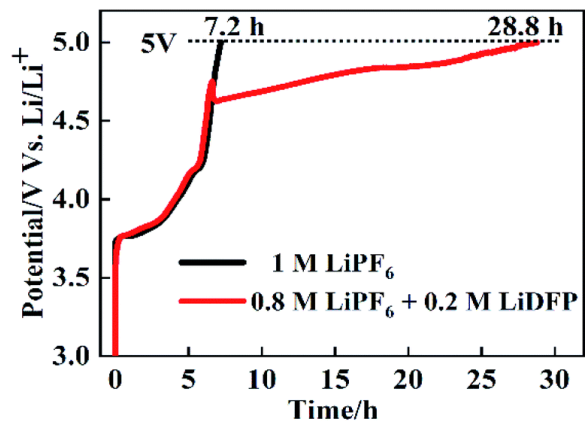
그림 51. LiPF 6 에 더해 LiPO 2 F 2 (LiDFP)를 추가했을 경우 과충전에 대한 문제도 일부 해결
