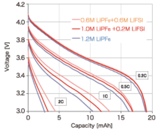
그림 47. -20°C의 저온에서 평가시 LiFSI 를 전해질로 첨가한 배터리의 방전 억제율이 LiPF 6 만 추가된 배터리 대비 향상
